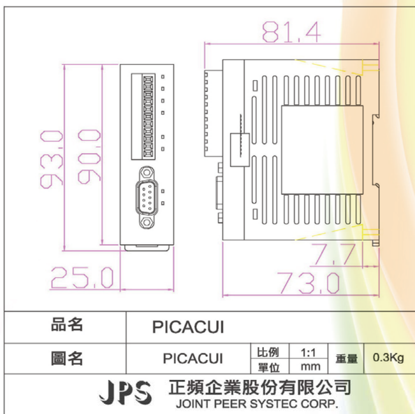
圖 1：PICACUI Unit：mm
