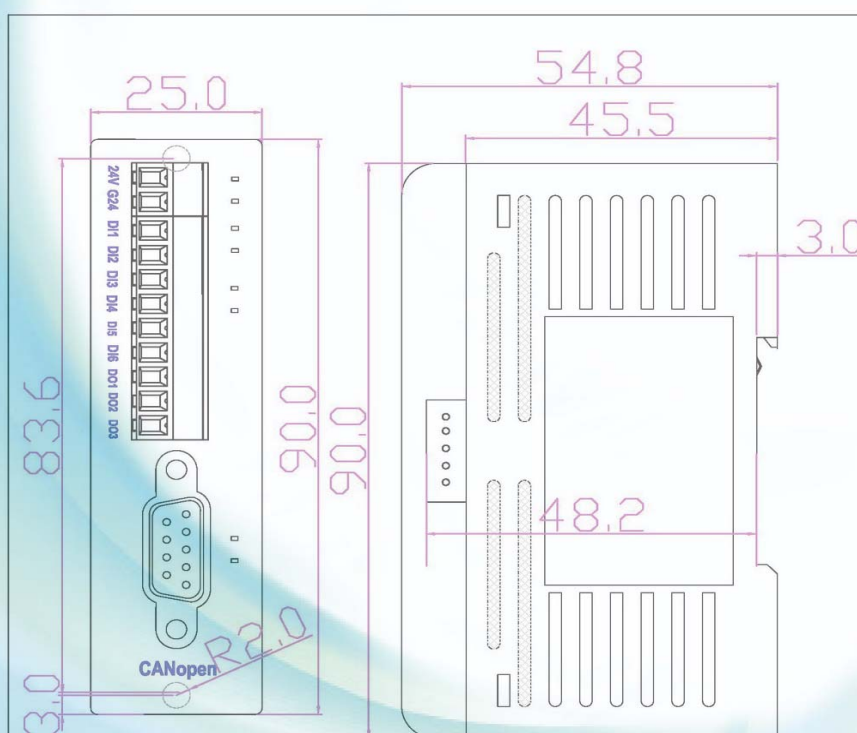
圖 1：CoMFIO Unit：mm
