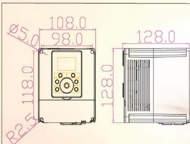
P1：馬力：0.5HP~2HP Unit：mm
