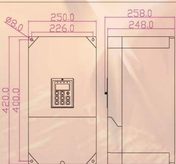
P4：馬力：15HP~30HP Unit：mm
