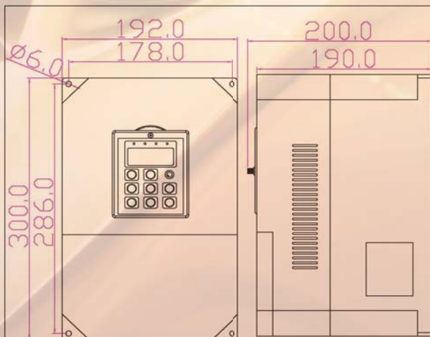
P3：馬力：7.5 HP~10HP Unit：mm
