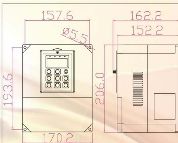
P2：馬力：3HP~5HP Unit：mm
