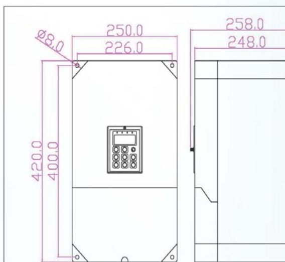
圖 4：馬力：15HP~30HP Unit：mm
