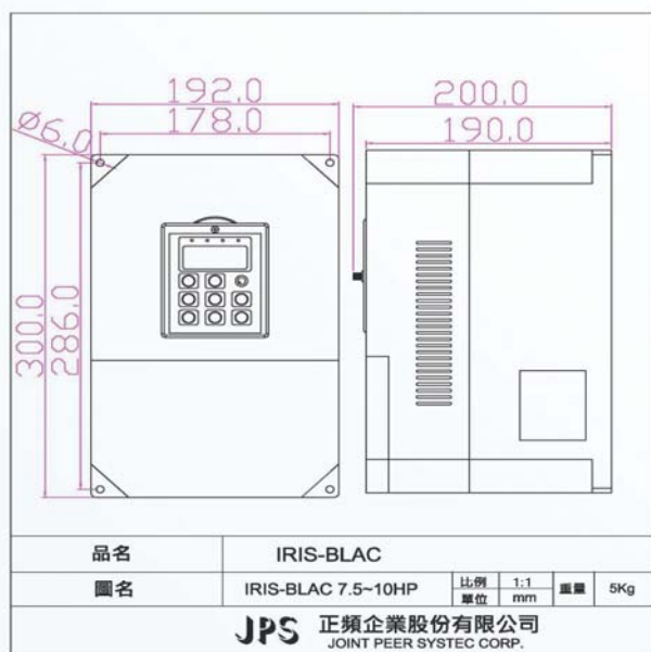
圖 3：馬力：7.5 HP~10HP Unit：mm
