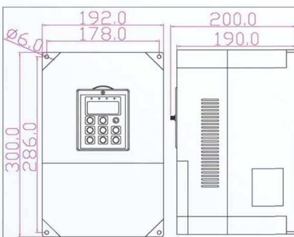
圖 3：馬力：7.5 HP~10HP Unit：mm
