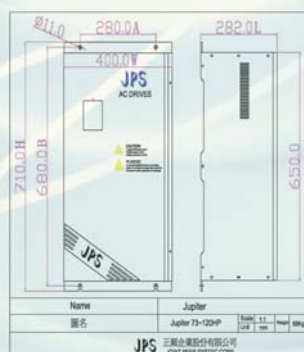
圖 6：馬力：73~120HP Unit：mm
