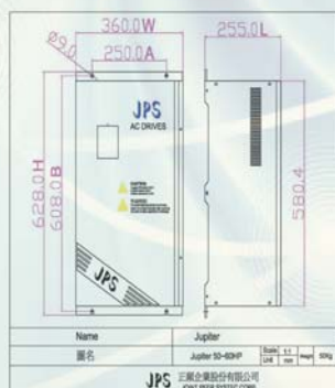
圖 5：馬力：50HP~60HP Unit：mm
