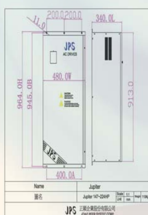
圖 7：馬力：147HP~224HP Unit：mm
