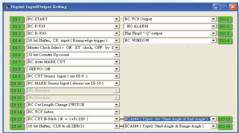
I/O 功能設定圖
