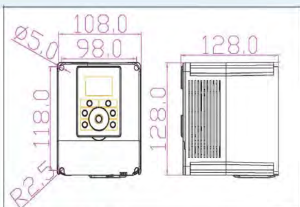
圖 1：馬力：05HP~2HP Unit：mm
