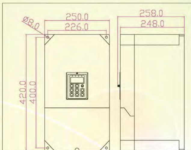
圖 4：馬力：15HP~30HP Unit：mm
