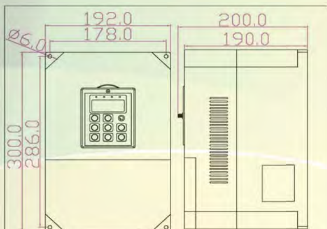
圖 3：馬力：7.5 HP~10HP Unit：mm
