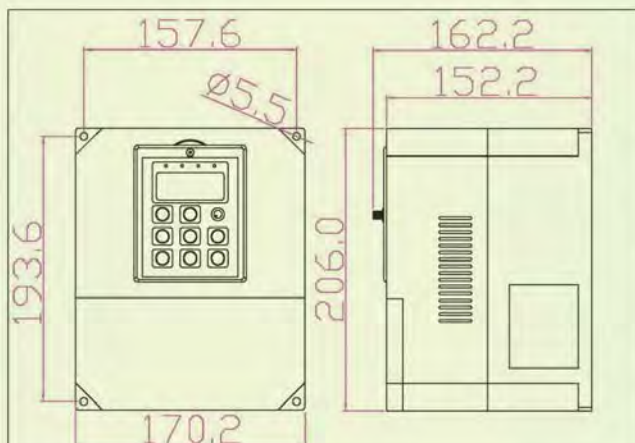
圖 2：馬力：3HP~5HP Unit：mm
